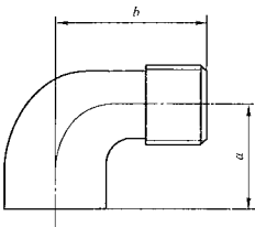
图 5 内外螺纹弯头 E4 表 7 内外螺纹弯头 E4 的尺寸
