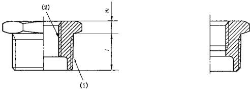
图 9 异径内外接头 B1
